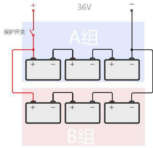
1KVA 2 组并接接线示意图
